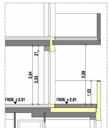
SNITT WOHNUNG - TERRASSE
