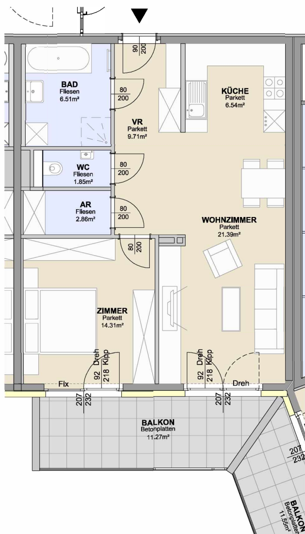
2. OBERGESCHOSS
