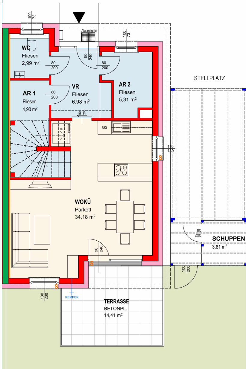
ERDGESCHOSS
