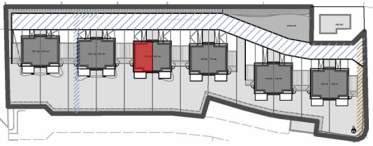
ÜBERSICHTSPLAN
