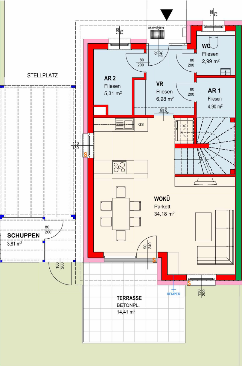
ERDGESCHOSS
