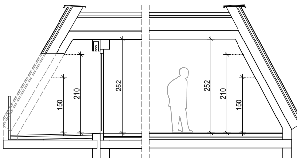
Systemschnitt M 1:100
