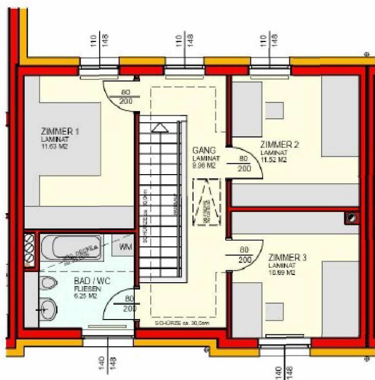
OBERGESCHOSS
