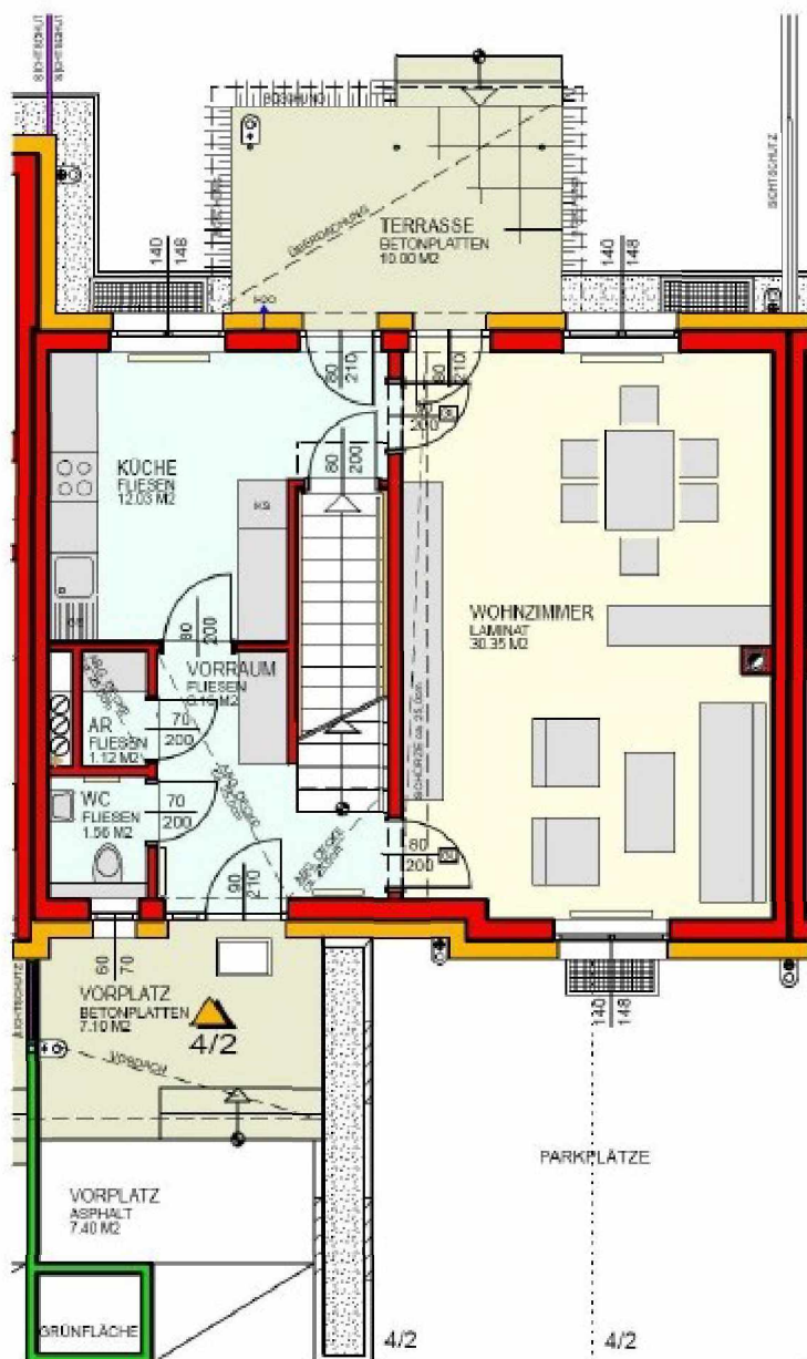
ERDGESCHOSS
