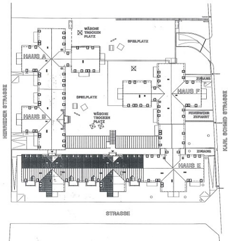
MELK XV 2. BAUSTUFE HAUS C und D GESAMTE WOHNHAUSANLAGE LAGEPLAN M 1 : 500
