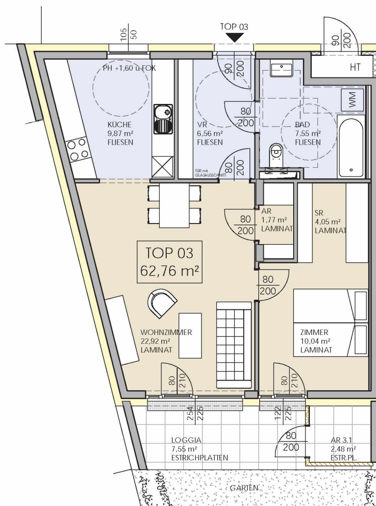
GRUDDRIS MIT MöBLIERUNGSVORSCHLAG
